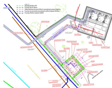
Projet de création d'une unité d'injection de nitrate de calcium et d'installation d'un groupe électrogène sur le PR Marina
