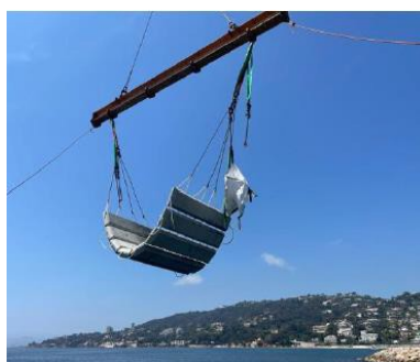
Travaux de réfection des matelas de stabilisation de l'émissaire de la STEP de Vallauris
